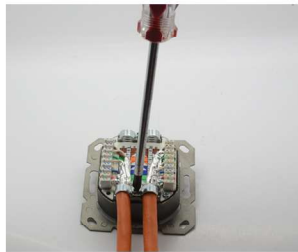
Selle für Abschirmung festziehen Tighten screen clamp
